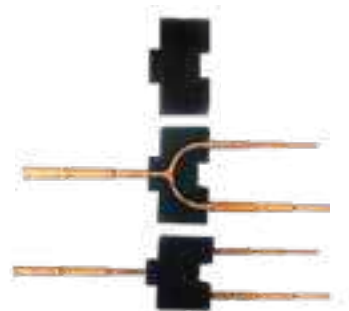
Refnet que não necessita brasagem BHRG25/26A33/72/73T
